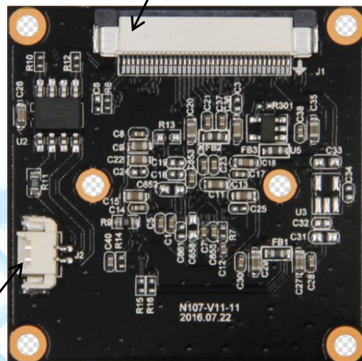
SENSOR 板反面
